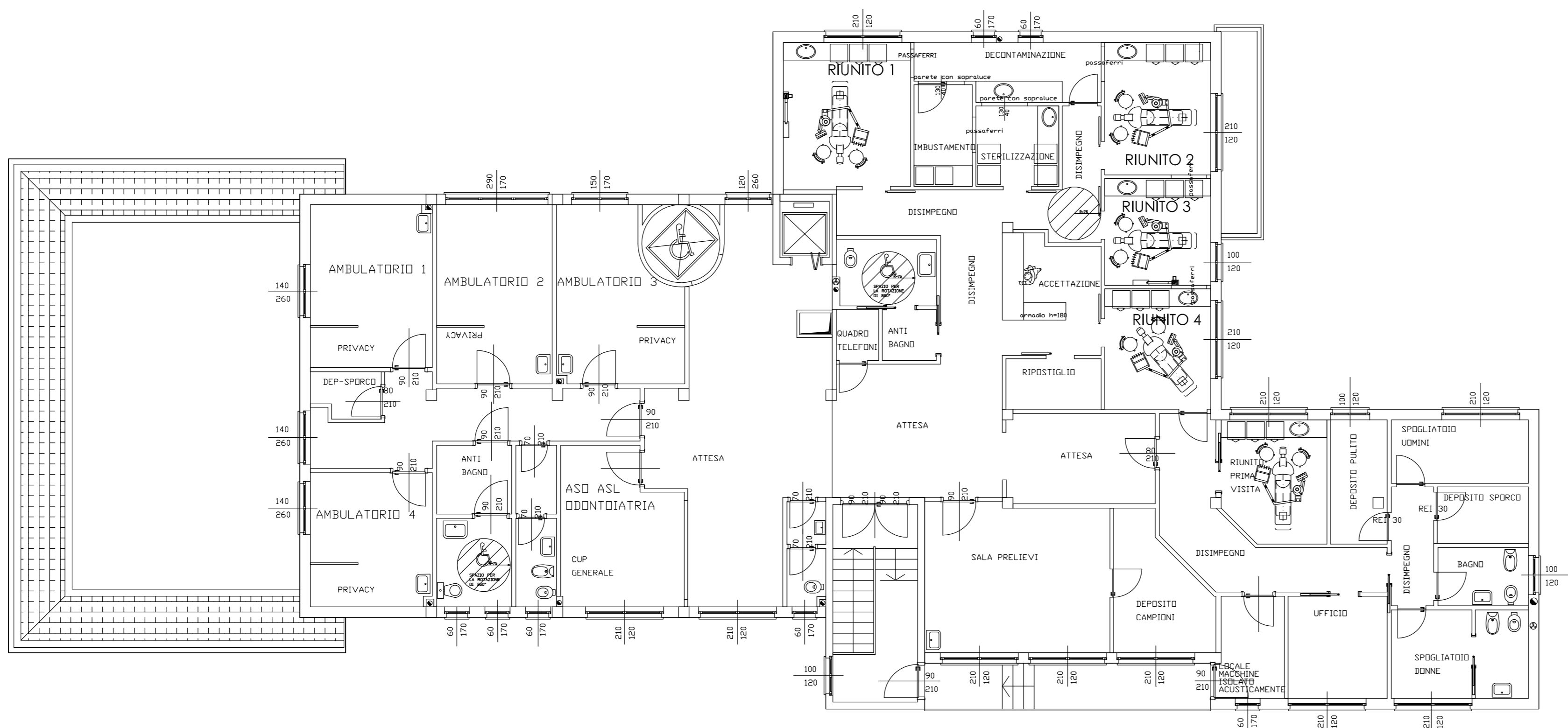
PIANO PRIMO
