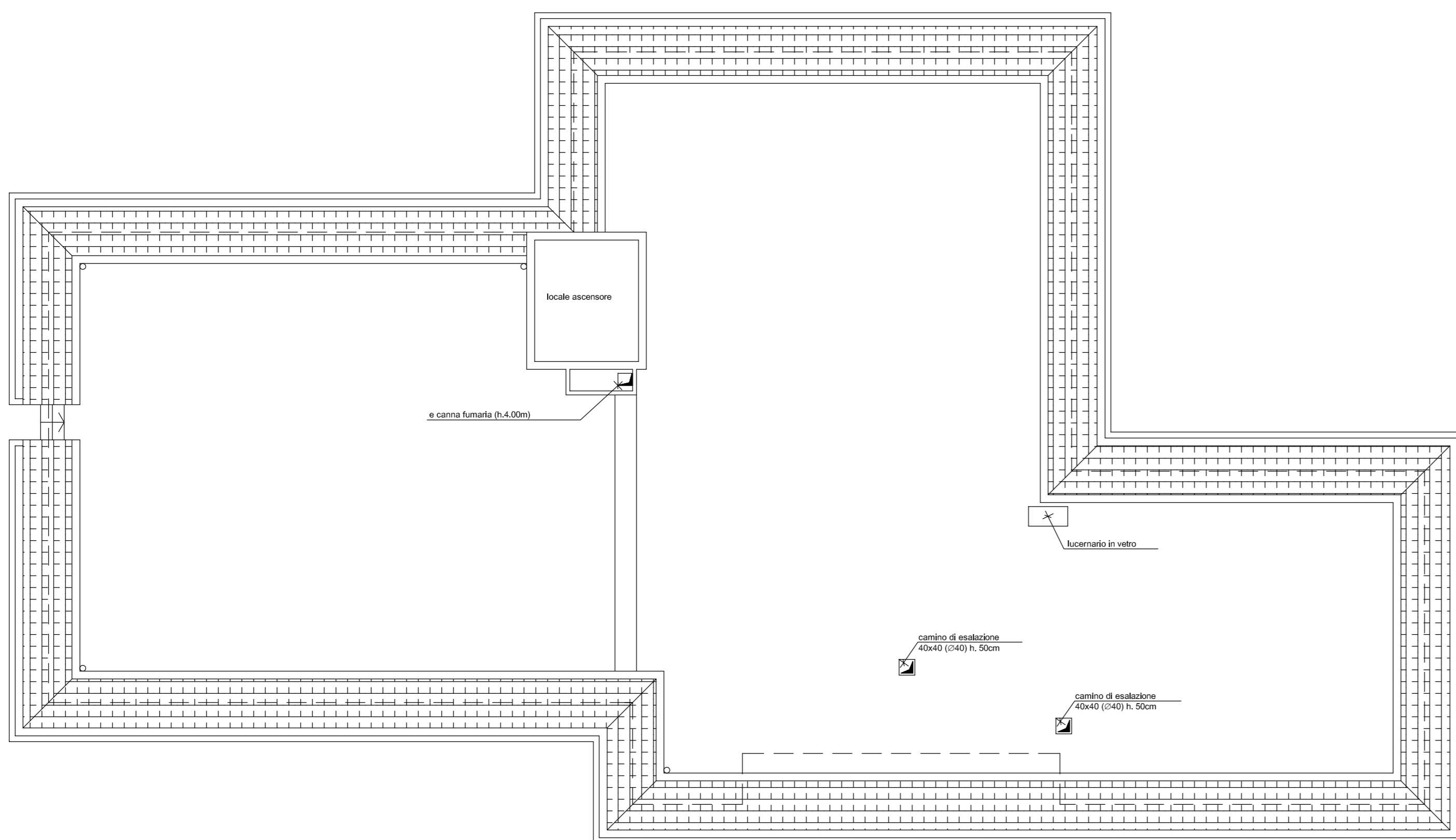
PIANO COPERTURA
